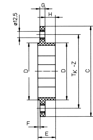
CF-K-100-125-150 Universal flange Elastikelement
